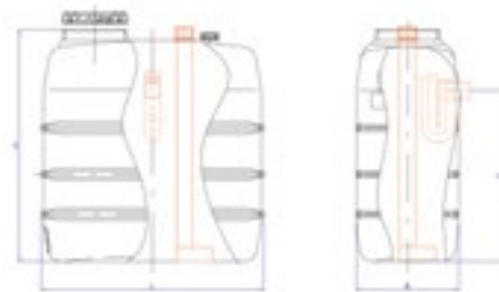
Basistank mit beruhigtem Zulauf und Überlaufsiphon
